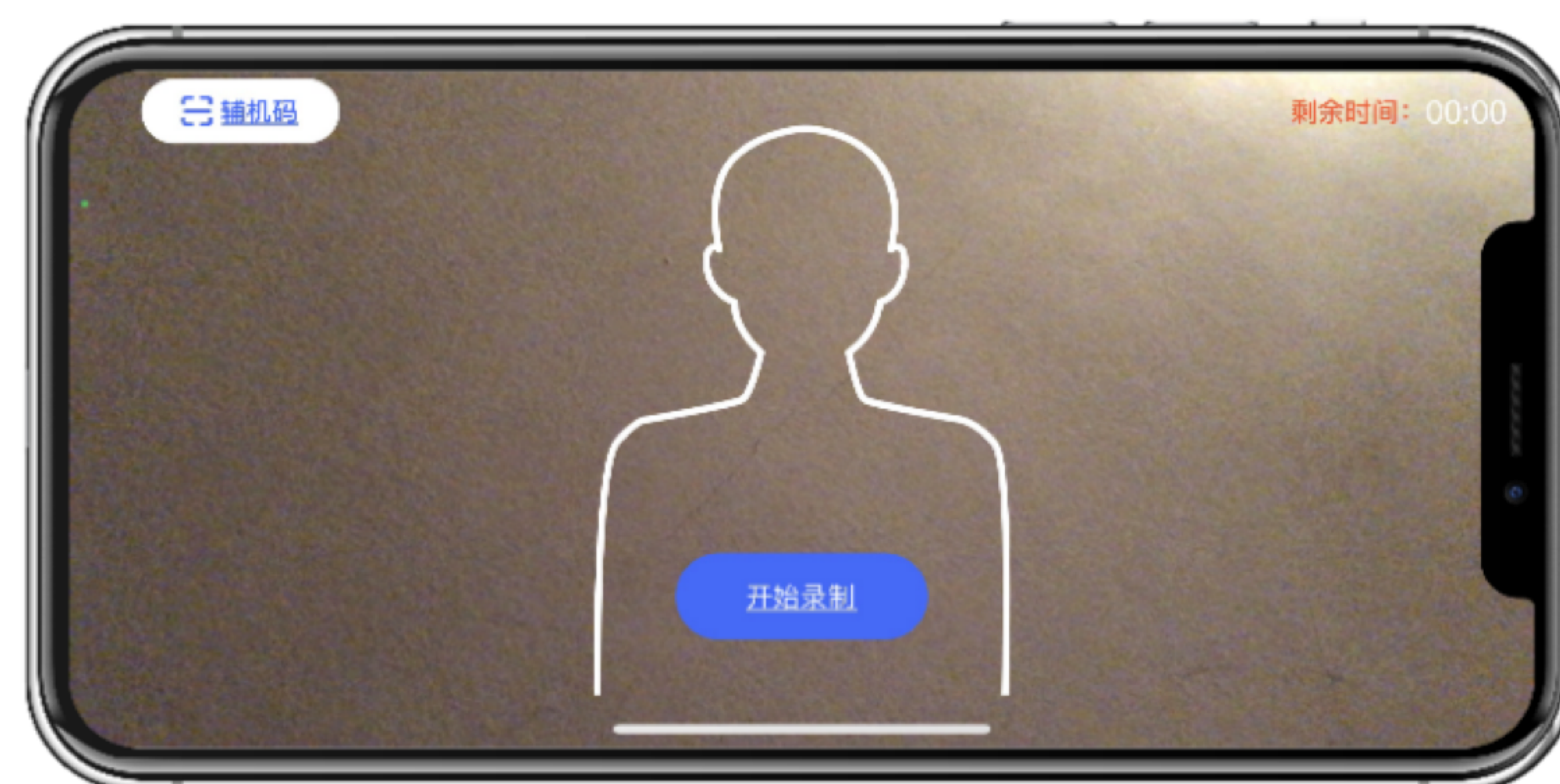
(图 20: 开始录制)
